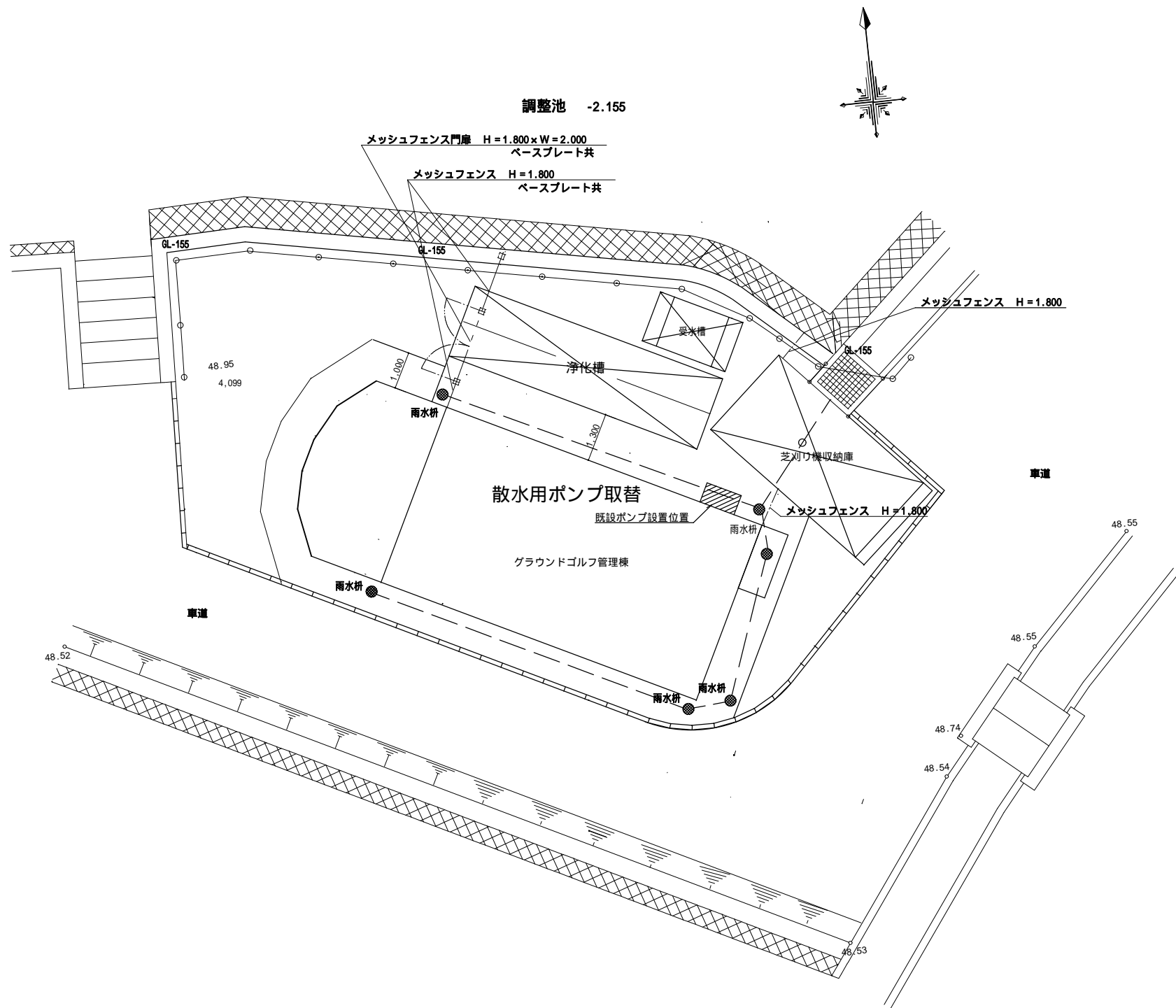
配置図 S:1/100
