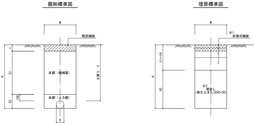
撤去工（石綿セメント管）
