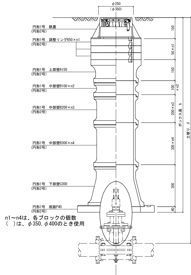
下部壁Cを使用する場合
