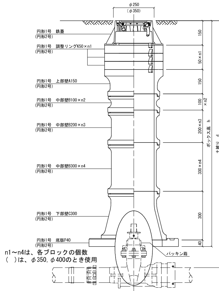
下部壁Cを使用する場合
