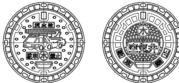
鉄蓋レイアウト例
