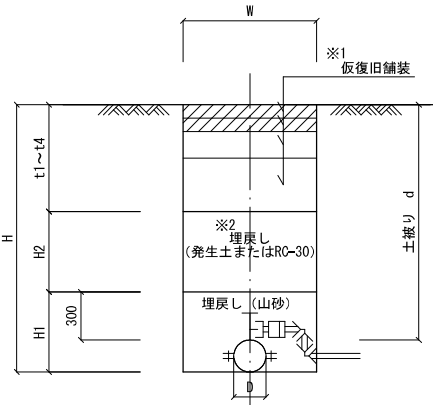
分岐部土工断面寸法表
