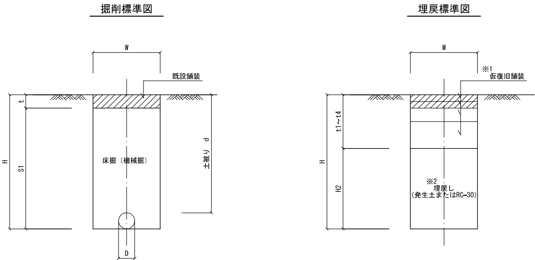
撤去工（石綿セメント管以外）
