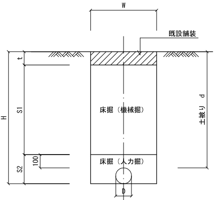
床掘断面図A-A'
