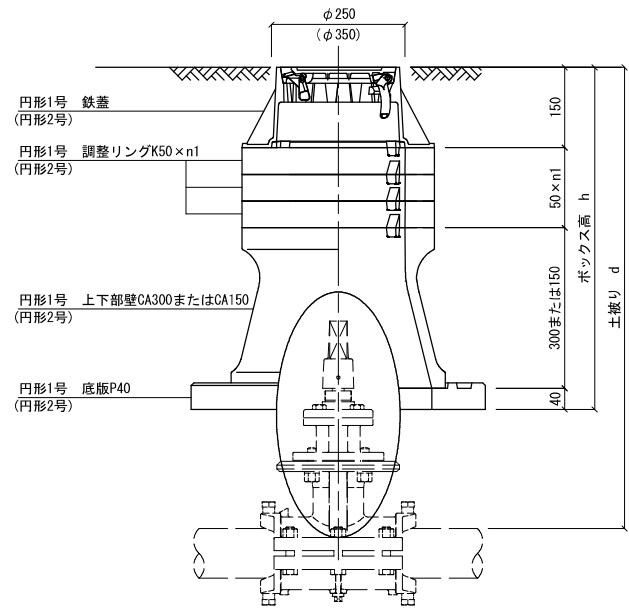
鉄蓋レイアウト例
