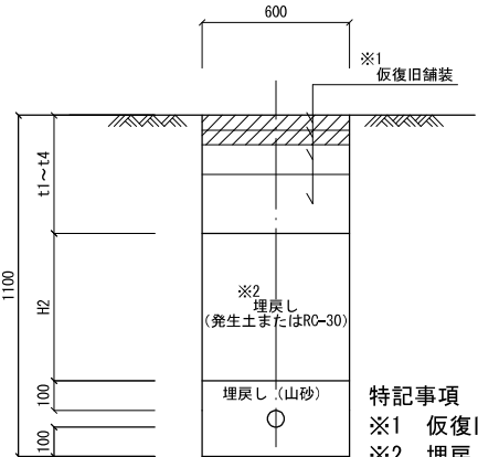
直線部土工断面寸法表
