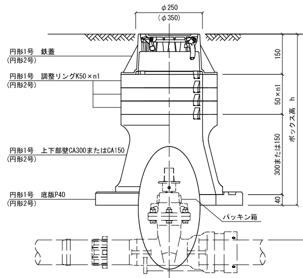
鉄蓋レイアウト例
