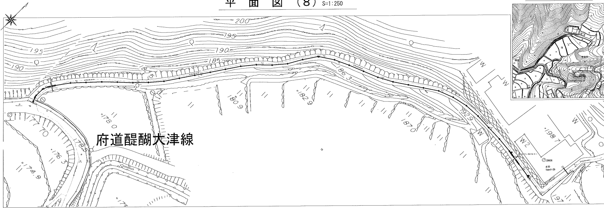
位置図 S=1:2,500
