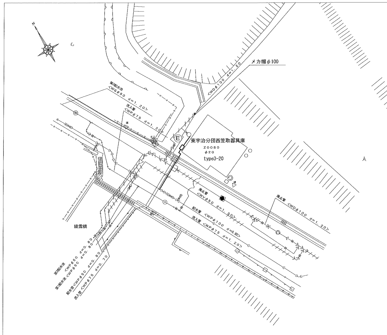
平面図 (5) 消防 S=1:100
