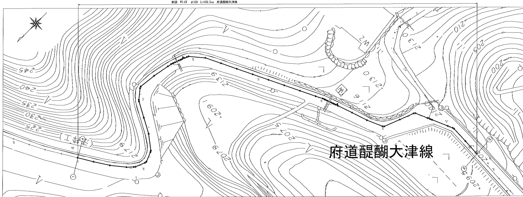
配管詳細図 (2) S=1:100
