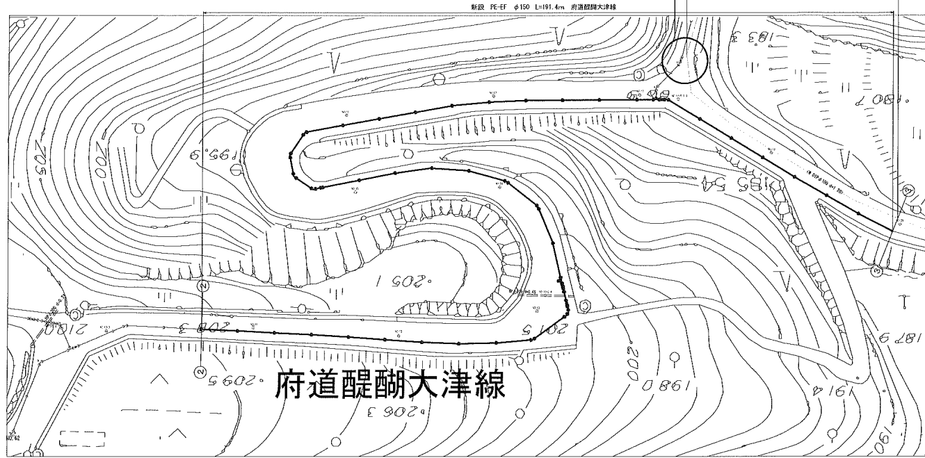
平面図 (3) S=1:250
