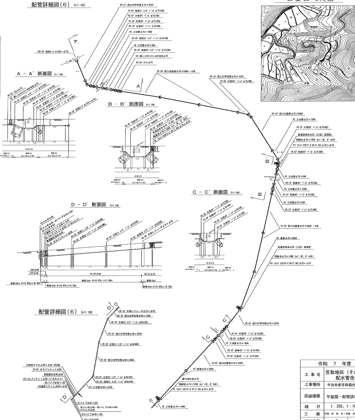
配管詳細図(6) S=1:100
