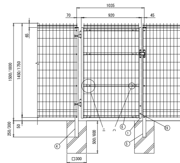
組立図 吊元が左、表開き (1/25)
