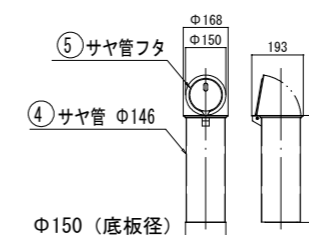
サヤ管詳細図
