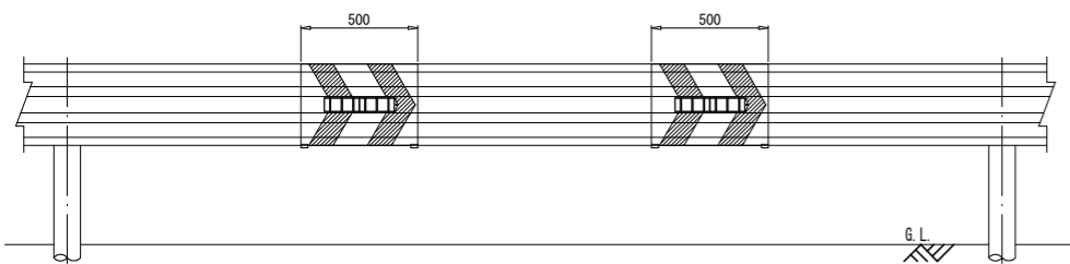
設置図 S=1/25
