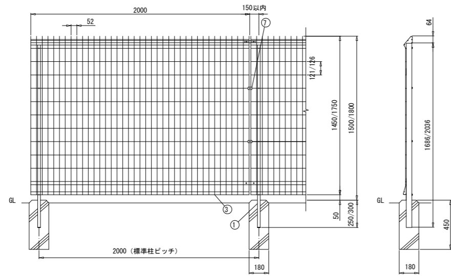
組立図 (1/25)
