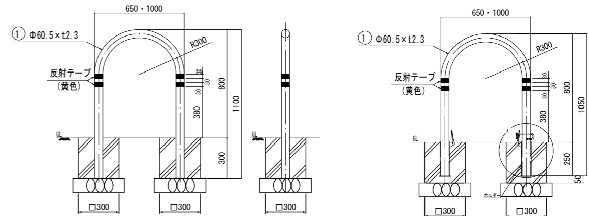
A部詳細図 (1/10)
