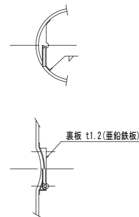
反射板取付部詳細図
