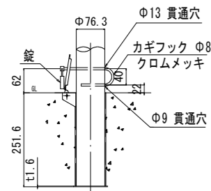
A部詳細図 (1/10)
