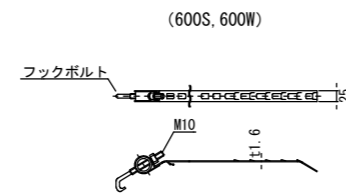
⑧ 取付バンド詳細図
