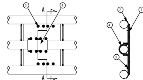
裏面図 S=1/10
