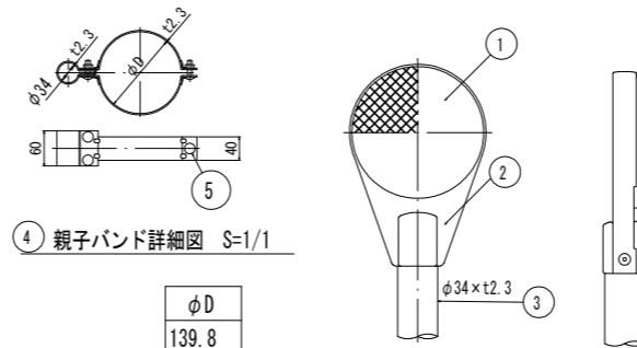
反射部詳細図 S=1/5
