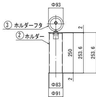
ホルダー詳細図 (1/10)
