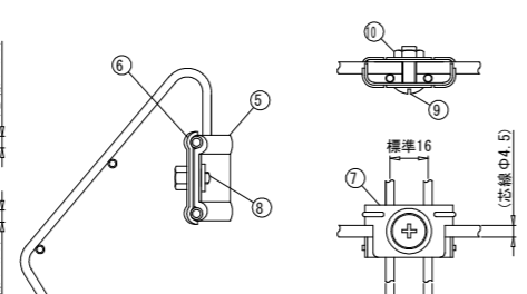
パネル止金具詳細図 (non scale) 注) パネル止金具の取付けは、逆方向(内側)からも可。
