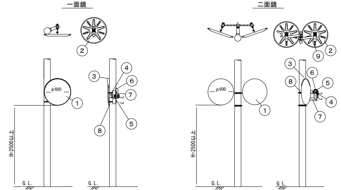
設置例 (2)
