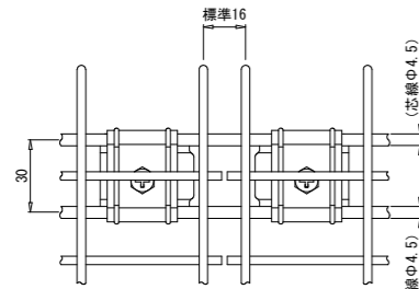
接続部詳細図 (non scale) 注) 接続金具の取付けは、逆方向(内側)からも可。
