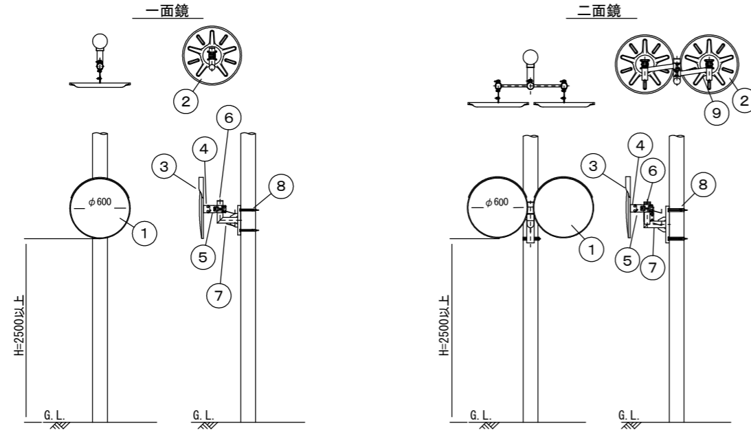
設置例 (1)
