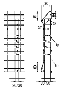
取付部詳細図 (non scale)
