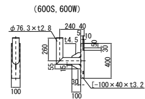
⑦ 電柱取付金具詳細図
