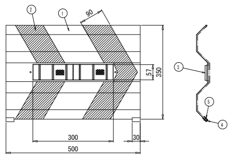
設置図 S=1/10
