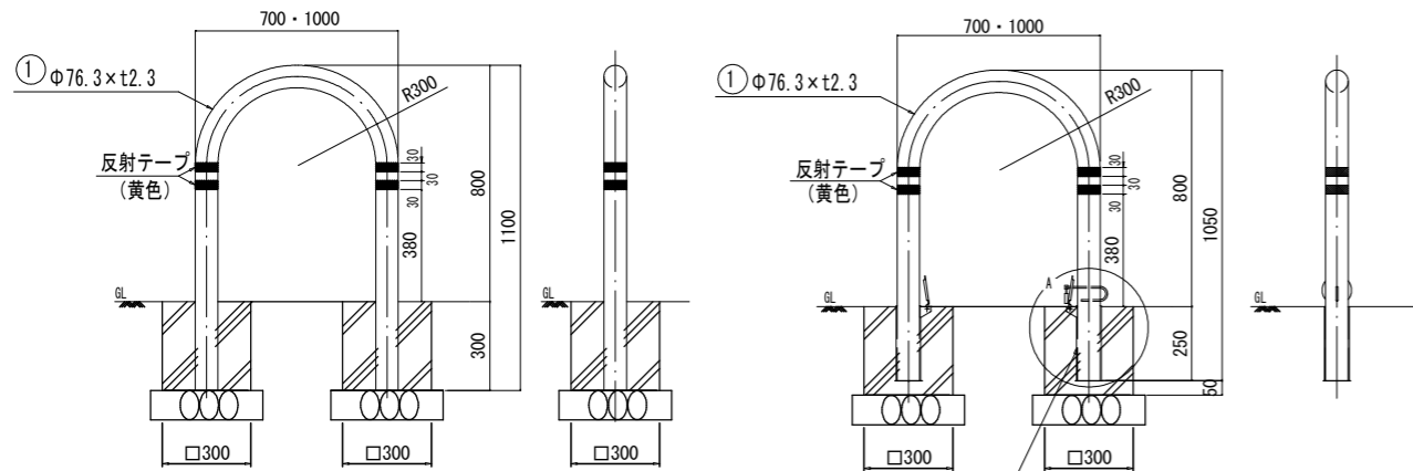
A部詳細図 (1/10)
