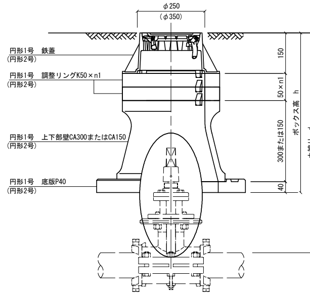
鉄蓋レイアウト例
