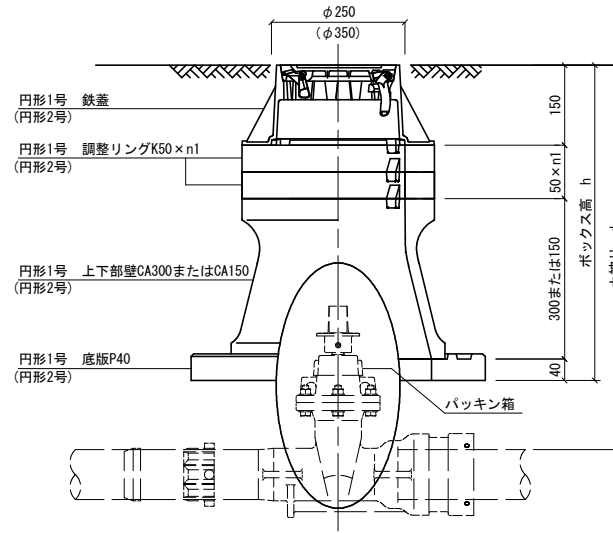
鉄蓋レイアウト例
